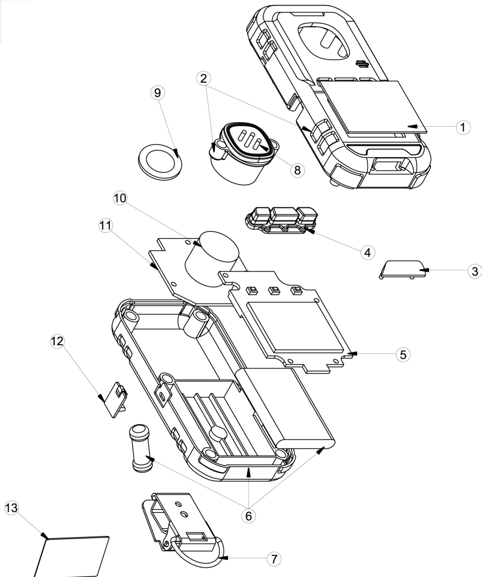
Рисунок 16 - Схема запасных частей
